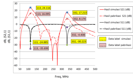
Gambar 10. Perbandingan hasil simulasi dan pengukuran rangkaian co-design dual band LNA dan BPF
