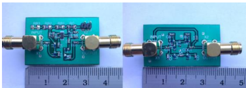
Gambar 9. Hasil Fabrikasi rangkaian dual band LNA (kiri) dan dual BPF (kanan)
